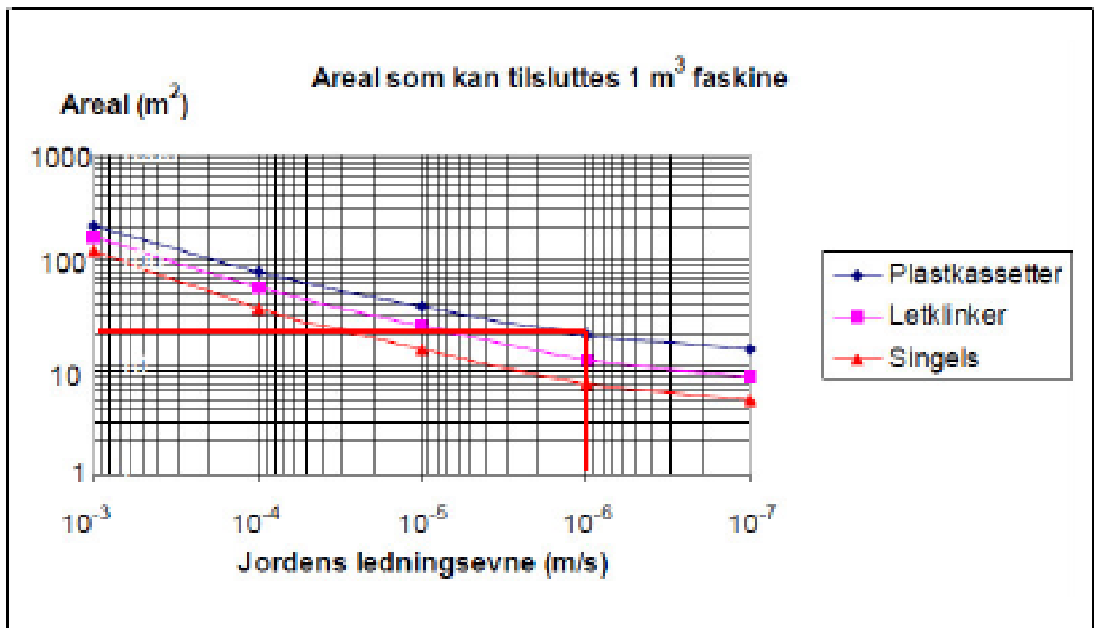
(Figur 2: Ud fra den beregnet ledningsevne, kan du ud fra ovenstående skema se, hvor stort et areal du kan tilslutte per 1 m³ faskine. Den tykke røde strg er eksemplet, der er vidst i følgende tekst)
