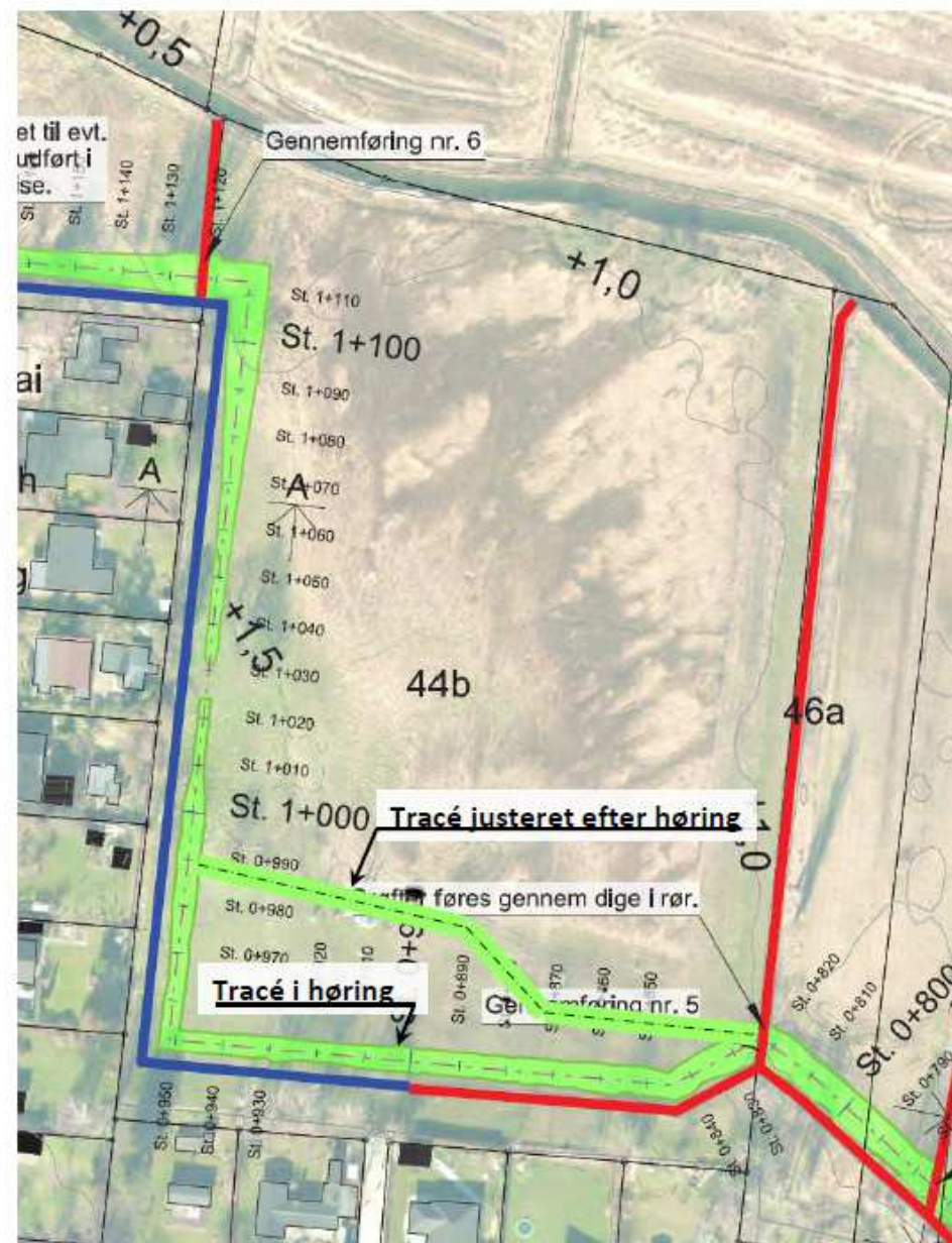
Østdige Justeret i forhold til høringssvar – inkl. Digelagets ønske om udretning
