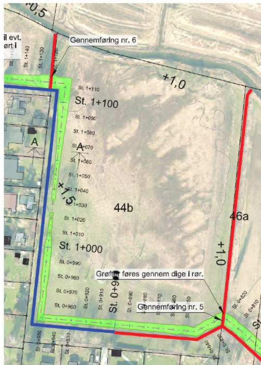
Justeret ØSTDige – i høring 06-10 til 06-11-2017
